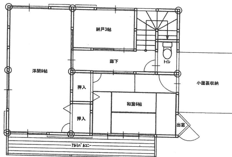
2階 平面図
